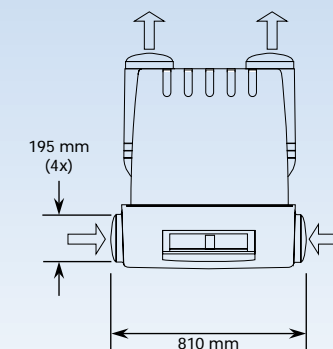
Mått Statiflex 200-M
